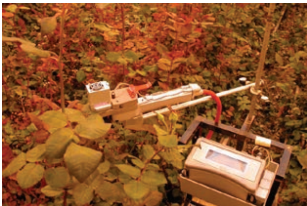
Figuur 1. Metingen met een draagbare fotosynthesemeter aan verschillende gewassen in de kas.
