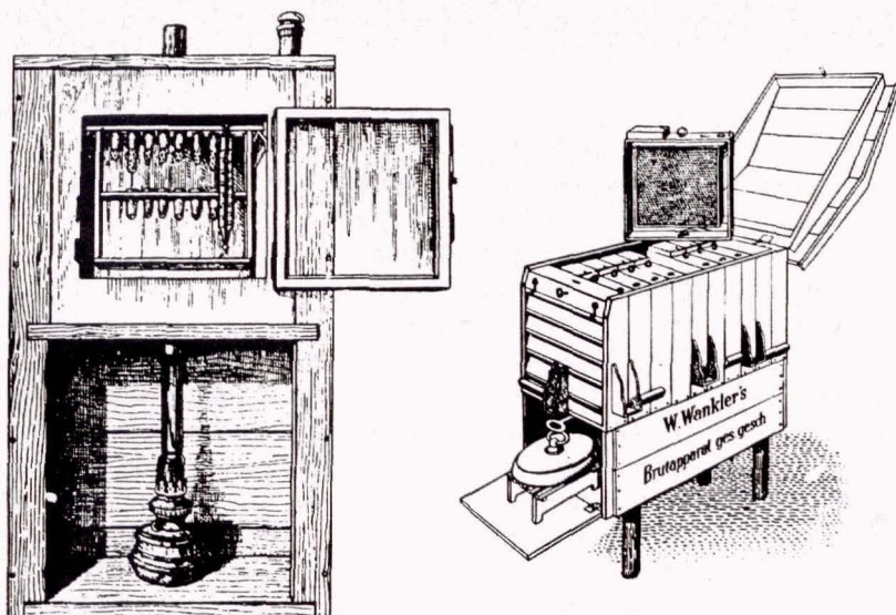
Abb. 3. Brutapparate nach Wankler (1924), links mit Petroleumlampe, rechts mit Wärmflasche
