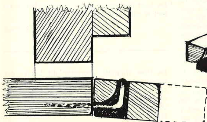
Spaarkast vliegplank aan schroefduim.
