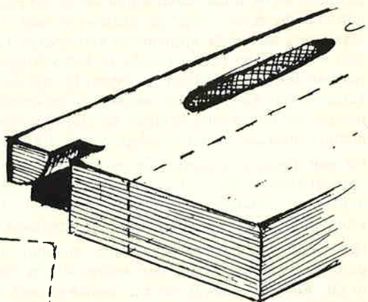
Vliegplank met oortje voor schroefduim, en sleuven voor transport ventilatie afgedekt met vliegengaas.
