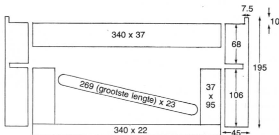
Vormdelen, dikte 20 mm, ter bevestiging op de basisplaat.
