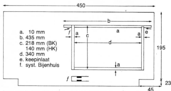
Basisplaat, dikte 20 mm; modelraampje ingetekend.
